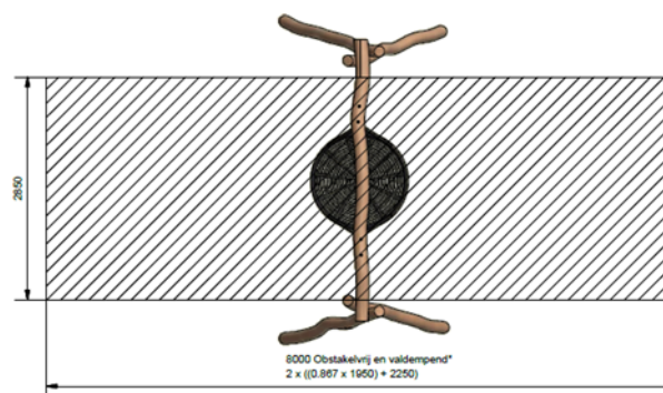
Veilige ruimte ( 1:50 ) Standaard plaatsing (valhoogte max 165 cm) Obstakelvrije ruimte dient geheel vrij te zijn van obstakels. Ondergrond minimaal geschikt voor een valhoogte van 165 cm
