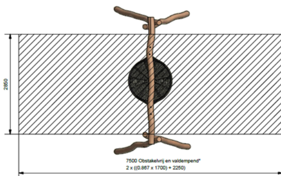
Veilige ruimte ( 1:50 ) Plaatsing op gras (valhoogte max 150 cm) Obstakelvrije ruimte dient geheel vrij te zijn van obstakels. Ondergrond minimaal geschikt voor een valhoogte van 150 cm (gras, zandondergrond)
