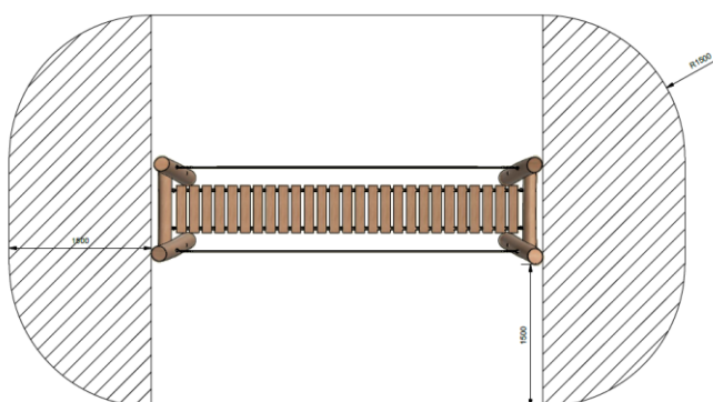
Obstakelvrije Zone ( 1 : 30 ) Obstakelvrije zone dient vrij te zijn van obstakels! Het materiaal van de ondergrond dient geschikt te zijn voor de valhoogte van het toestel!"
