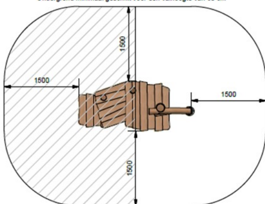
Plaatsing in vrije ruimte (1:50) Obstakelvrije ruimte dient geheel vrij te zijn van obstakels* Ondergrond minimaal geschikt voor een valhoogte van 60 cm
